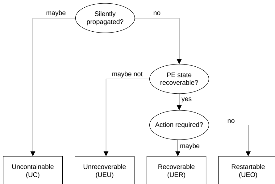
Figure D10-1 PE error states
