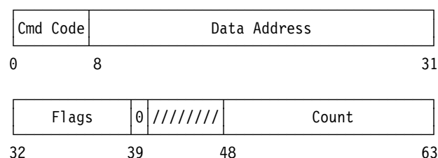
Format-1 CCW
