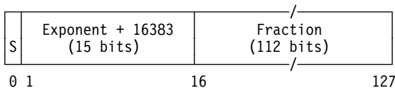
Figure 19-6. BFP Extended Format (16 bytes)
