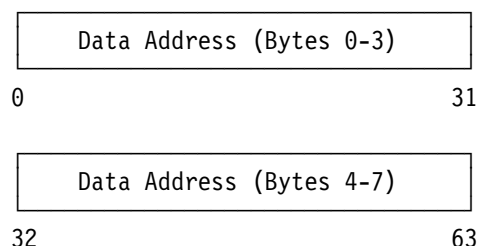
Format-2 IDAW
