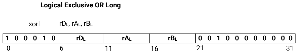
Figure 194: xorl
