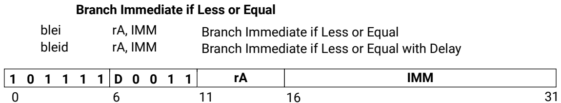
Figure 72: blei
