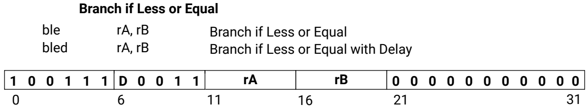
Figure 71: ble
