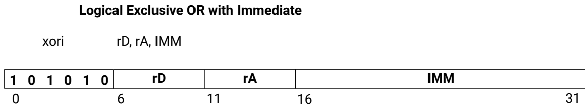
Figure 144: xori
