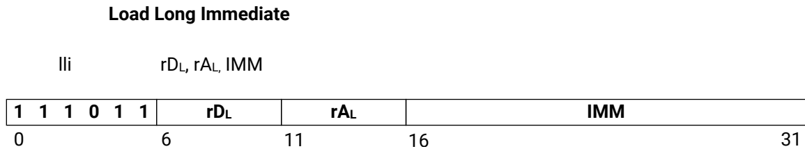
Figure 178: lli
